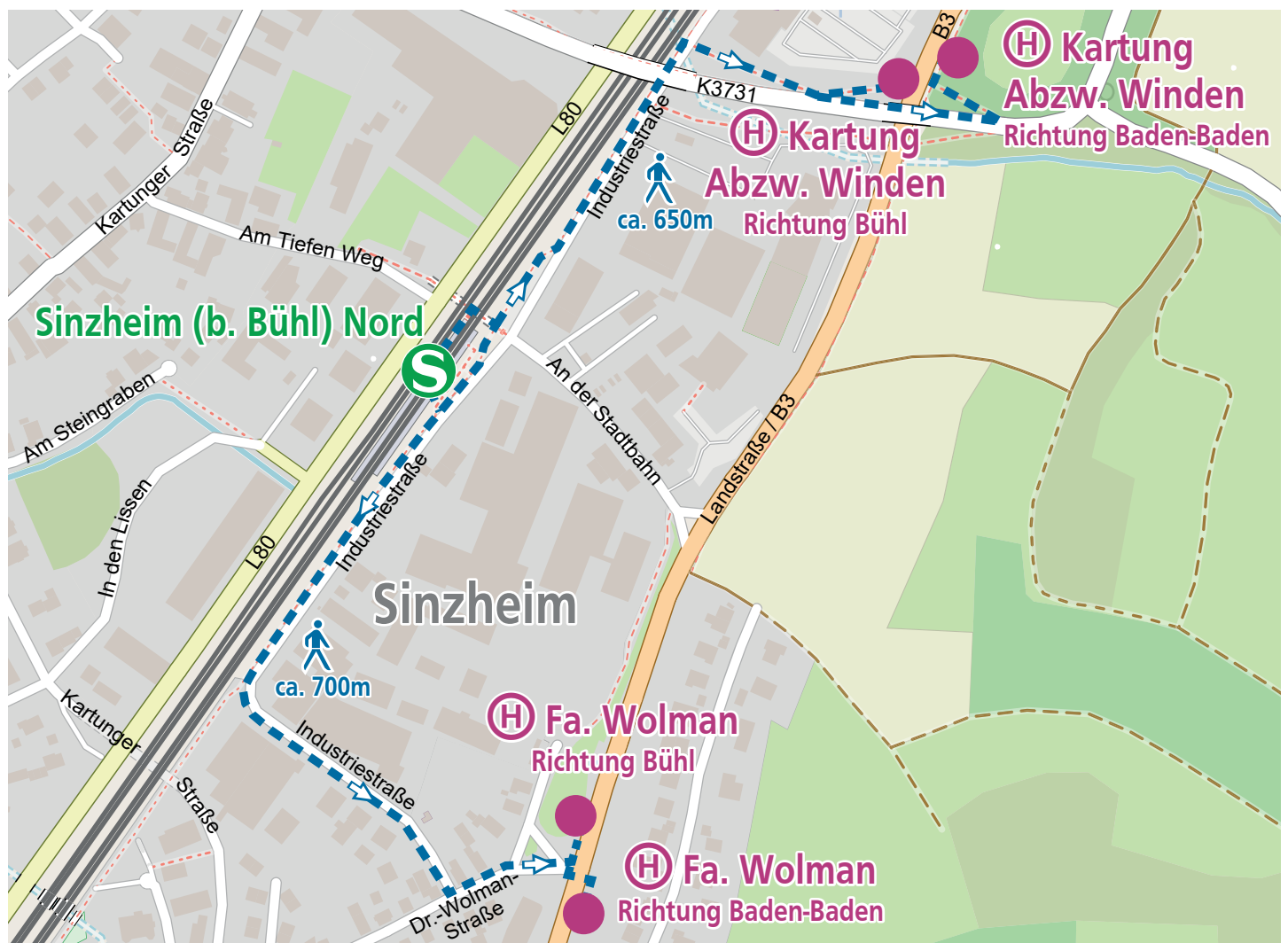
Kartgrundlage: OpenStreetMap-Mitwirkende
